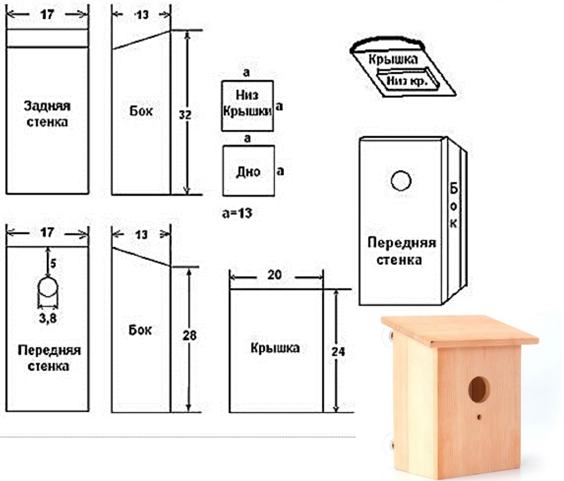
Чертеж 2. «Скворечник с двухскатной крышей»
